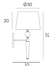
1G1517 C GO E27 max 60W
