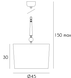
1G1618 C GO E27 max 60W
