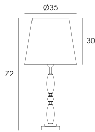
1G1202 C GO E27 max 60W
