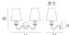
1G2204 C GO E27 max 60W
