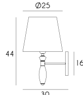
1G1503 C GO E27 max 60W
