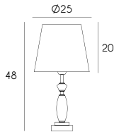
1G1101 C GO E27 max 60W
