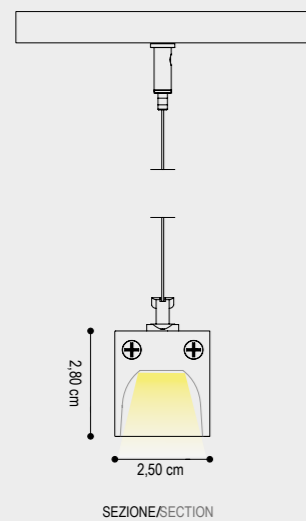
LA SOSPENSIONE RIGALED PREVEDE L'INSTALLAZIONE DELL'OTTICA ARRETRATA THE RIGALED SUSPENSION PROVIDES THE INSTALLATION OF THE BACKGROUND OPTICS
