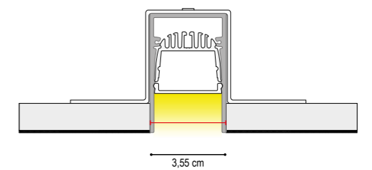
INSTALLAZIONE AD INCASSO LARGHEZZA TAGLIO L=3,55cm RECESSED INSTALLATION CUTTING WIDTH L=3,50 cm
