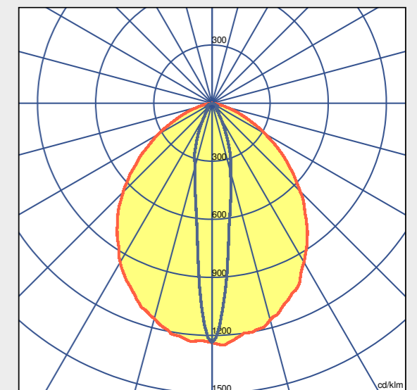
DIAGRAMMA FOTOMETRICO LENTE SPOT - 15°
