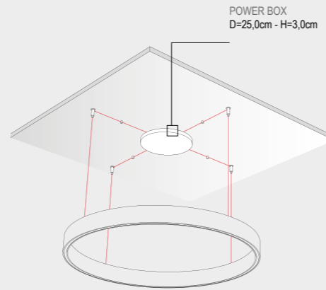
OLIMPIA CON BOX OLIMPIA WITH POWER SUPPLY BOX
