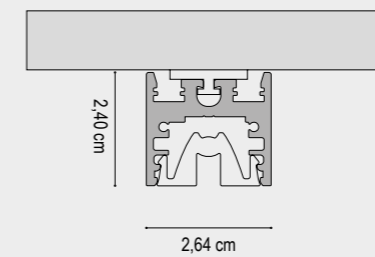
INSTALLAZIONE CON STAFFE MAGNETICHE SU SUPERFICIE METALLICA ORIZZONTALE INSTALLATION WITH MAGNET ON HORIZONTAL METAL SURFACE
