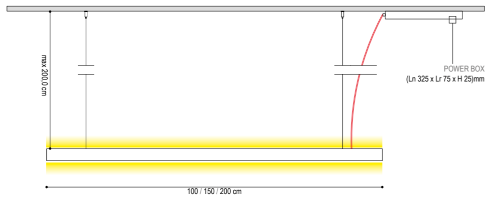
SEZIONE/SECTION
