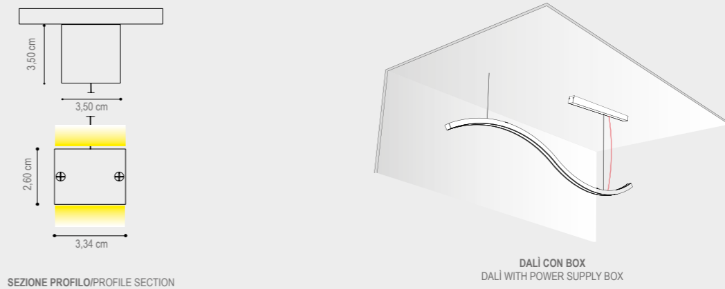
SEZIONE PROFILO/PROFILE SECTION
