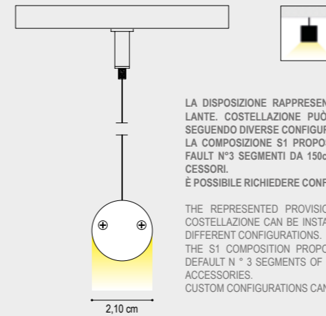
SEZIONE PROFILO/PROFILE SECTION
