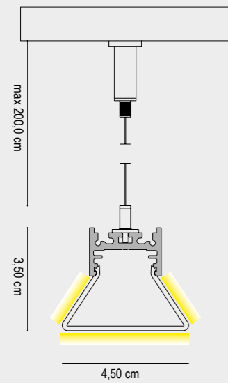
INSTALLAZIONE A SOSPENSIONE SUSPENSION
