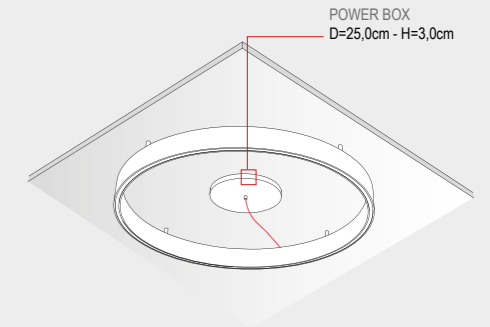
OLIMPIA CON BOX OLIMPIA WITH POWER SUPPLY BOX
