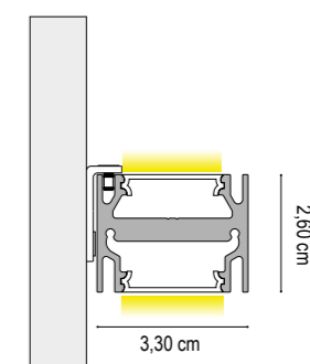
INSTALLAZIONE A PARETE WALL INSTALLATION
