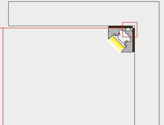
INSTALLAZIONE SU SUPERFICI ORIZZONTALI E VERTICALI INSTALLATION ON HORIZONTAL AND VERTICAL SURFACES
