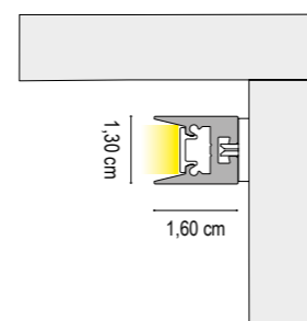
INSTALLAZIONE CON CLIP IN POLICARBONATO SU SUPERFICIE VERTICALE INSTALLATION WITH POLYCARBONATE CLIP ON A VERTICAL SURFACE
