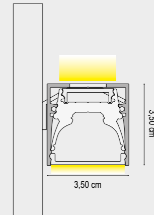
ZER035X-P CON DIFFUSORE ESTERNO ZER035X-P WITH EXTERNAL DIFFUSER
