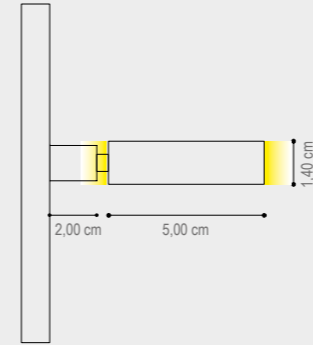
SEZIONE PROFILO/PROFILE SECTION
