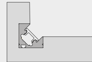
INSTALLAZIONE AD INCASSO RECESSED INSTALLATION
