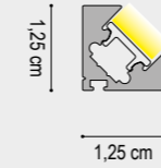
INSTALLAZIONE AD INCASSO RECESSED INSTALLATION
