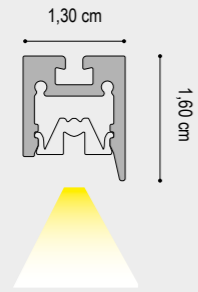
VERSIONE SPOT (15°) SPOT VERSION (15°)
