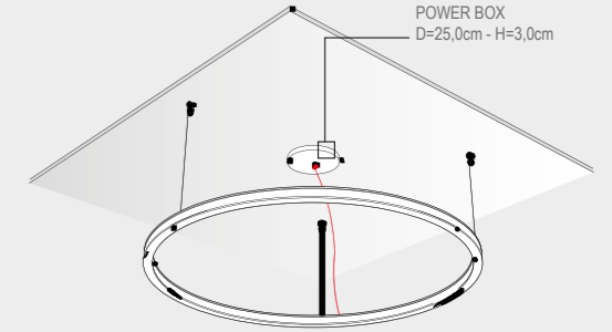
GIOTTO CON BOX GIOTTO WITH POWER SUPPLY BOX
