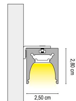
INSTALLAZIONE A PARETE WALL INSTALLATION
