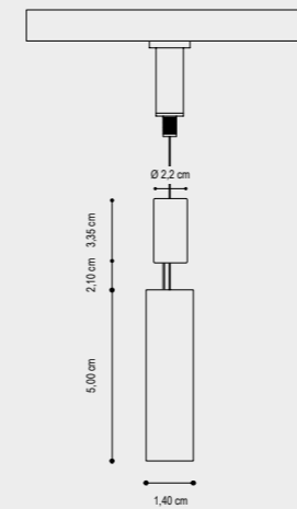
SEZIONE PROFILO/PROFILE SECTION
