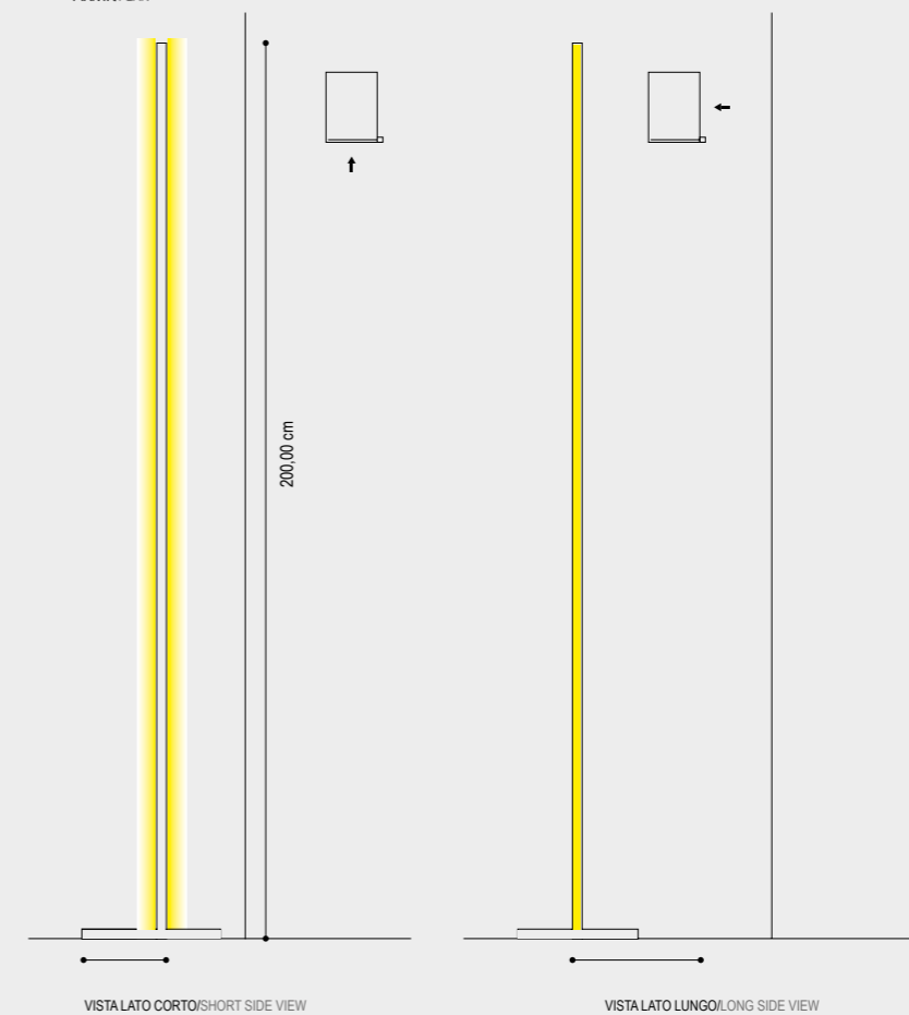
VISTA LATO CORTO/SHORT SIDE VIEW
