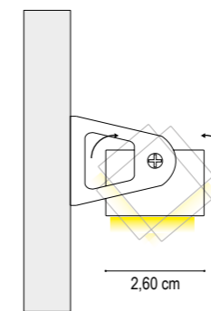
INSTALLAZIONE CON CLIP IN POLICARBONATO SU SUPERFICIE ORIZZONTALE INSTALLATION WITH POLYCARBONATE CLIP ON HORIZONTAL SURFACE
