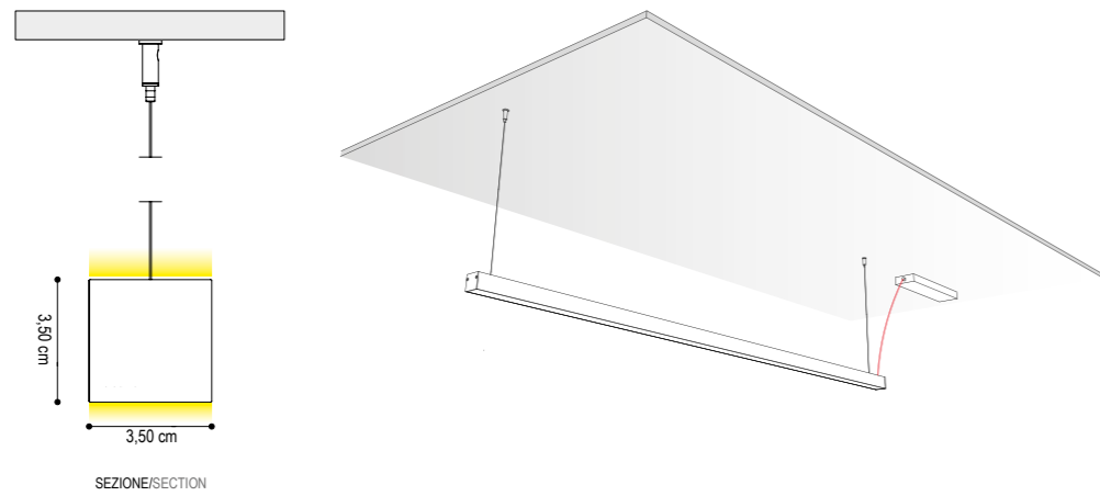
SEZIONE/SECTION
