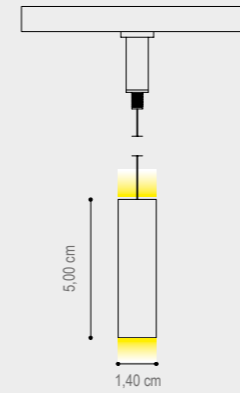
SEZIONE PROFILO/PROFILE SECTION
