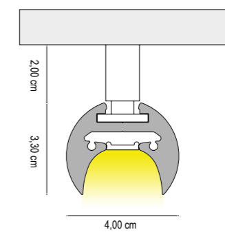
INSTALLAZIONE A SOFFITTO CON DISTANZIALE PRODOTTO MONOEMISSIONE CEILING INSTALLATION WITH SPACER MONO EMISSION PRODUCT
