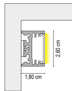
INSTALLAZIONE CON CLIP IN POLICARBONATO SU SUPERFICIE VERTICALE INSTALLATION WITH POLYCARBONATE CLIP ON A VERTICAL SURFACE
