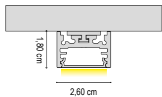
INSTALLAZIONE CON CALAMITA SU SUPERFICIE METALLICA ORIZZONTALE E VERTICALE INSTALLATION WITH MAGNET ON HORIZONTAL AND VERTICAL METAL SURFACE
