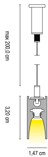
INSTALLAZIONE A SOSPENSIONE SUSPENSION
