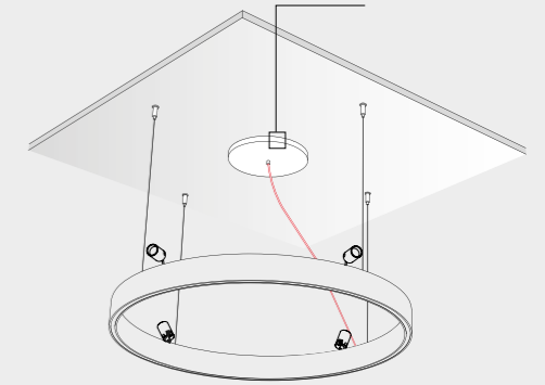
OLIMPIA CON BOX OLIMPIA WITH POWER SUPPLY BOX
