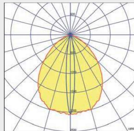
DIAGRAMMA FOTOMETRICO LENTE SPOT - 15°
