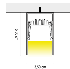
INSTALLAZIONE A SOFFITTO CEILING INSTALLATION
