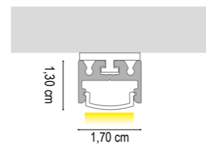
INSTALLAZIONE CON CALAMITA SU SUPERFICIE METALLICA ORIZZONTALE E VERTICALE INSTALLATION WITH MAGNET ON HORIZONTAL AND VERTICAL METAL SURFACE
