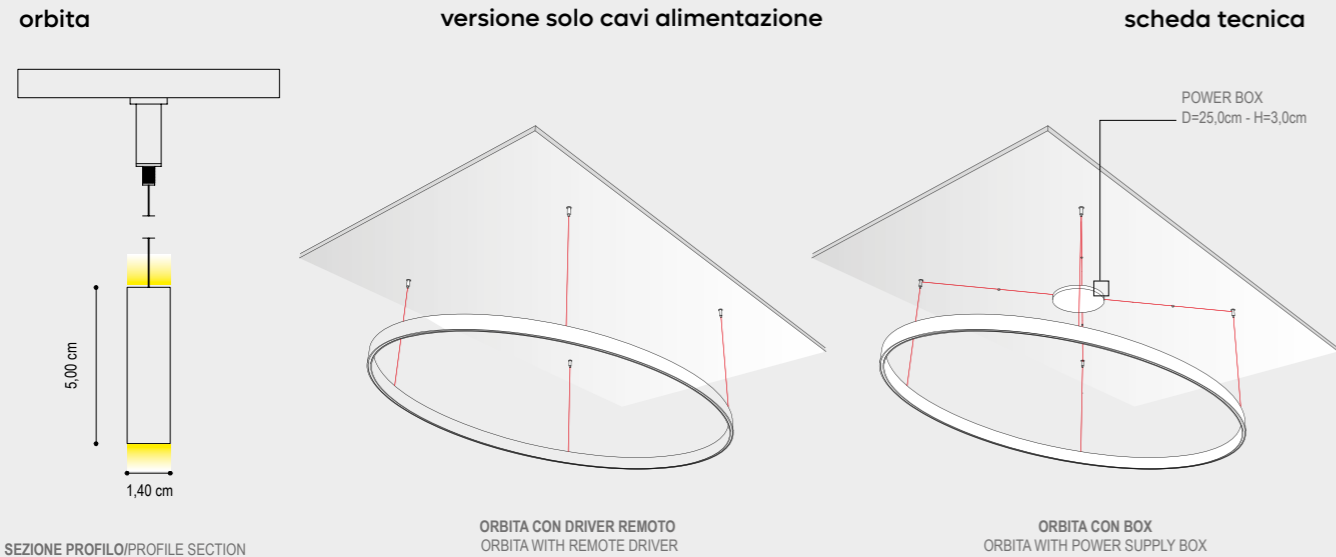
SEZIONE PROFILO/PROFILE SECTION
