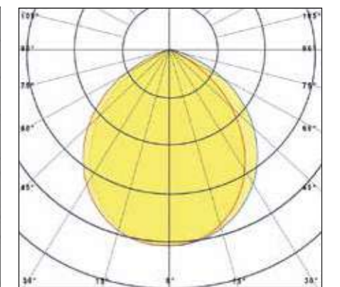
DIFFUSORE IN POLICARBONATO OPALE OPAL POLYCARBONATE DIFFUSER
