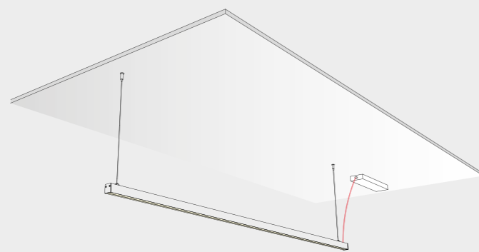
LA SOSPENSIONE RIGALED PREVEDE L'INSTALLAZIONE DELL'OTTICA ARRETRATA THE RIGALED SUSPENSION PROVIDES THE INSTALLATION OF THE BACKGROUND OPTICS
