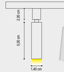
SEZIONE PROFILO/PROFILE SECTION
