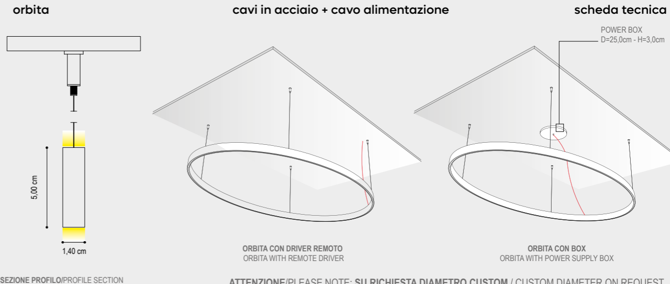
SEZIONE PROFILO/PROFILE SECTION
